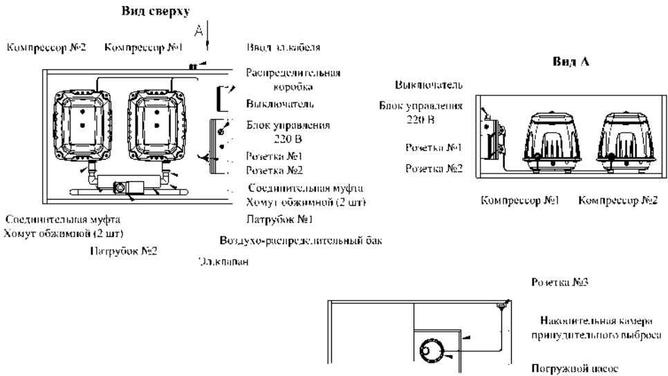
Рис. №6. УОСВ ТОПАС 40 - 50 с принудительным выбросом очищенной воды
