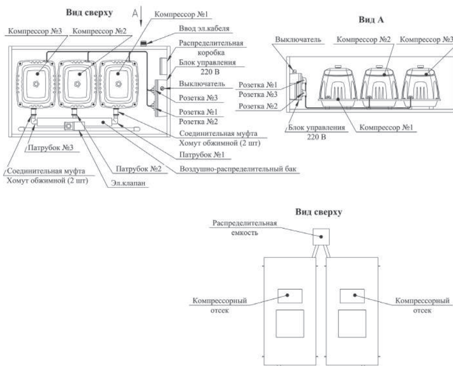
Рис. №11. УОСВ ТОПАС 150 с самотечным отводом очищенной воды
